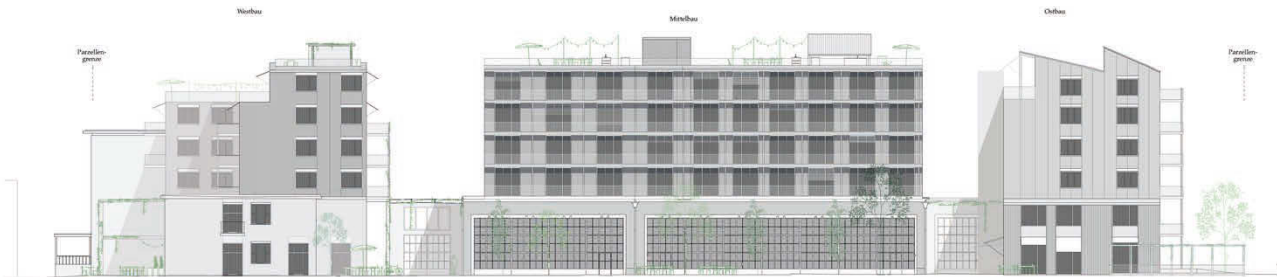
Ansicht Südwest
