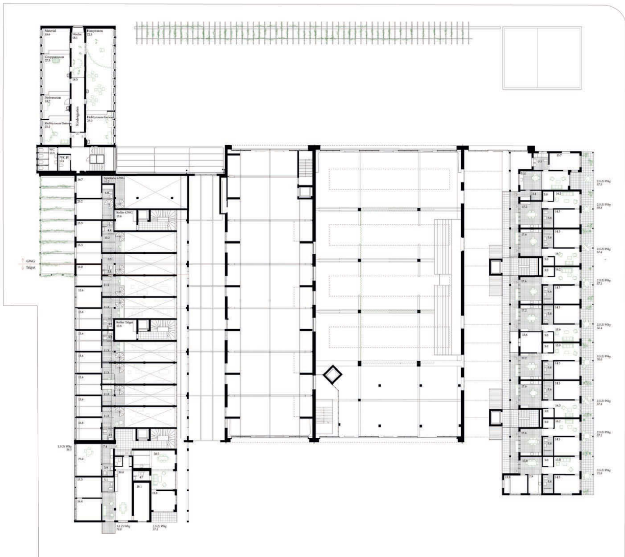
Grundriss 1. OG
