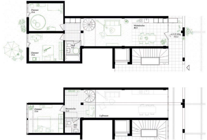
Westbau 4.5 Zi. Maisonette
