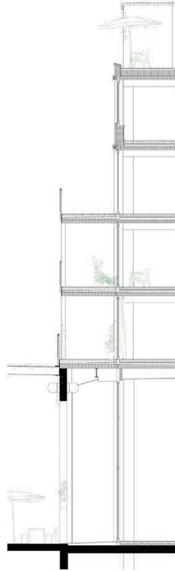
Detailschnitt C-C und Detailansicht des Westbaus, Wohnhaus an der Gewerbeasse
