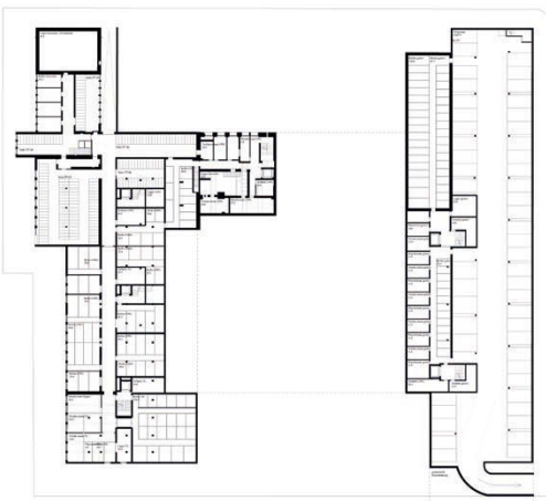
Grundriss UG
