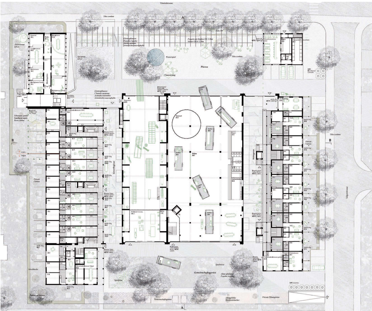
Grundriss EG
