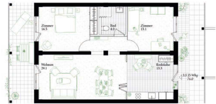
Westbau 3.5 Zi. Wohnung
