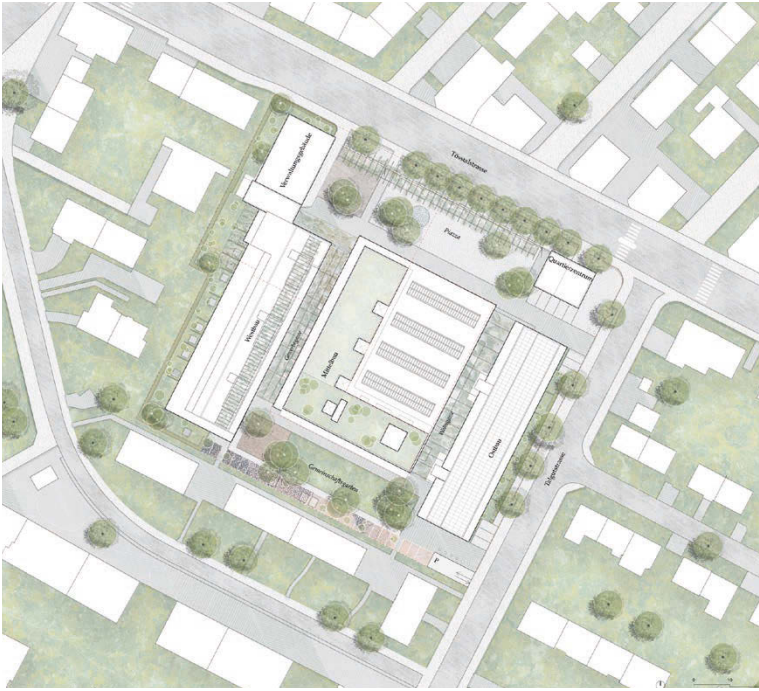
Situationsplan mit Dachaufsicht
